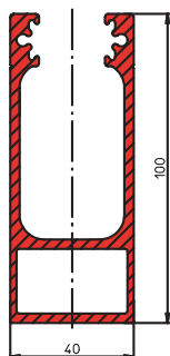
Styrskena (geider) 40 x 100 mm
